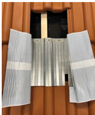
SDPV Grundträger rechts und links einlegen und flexibel anformen
